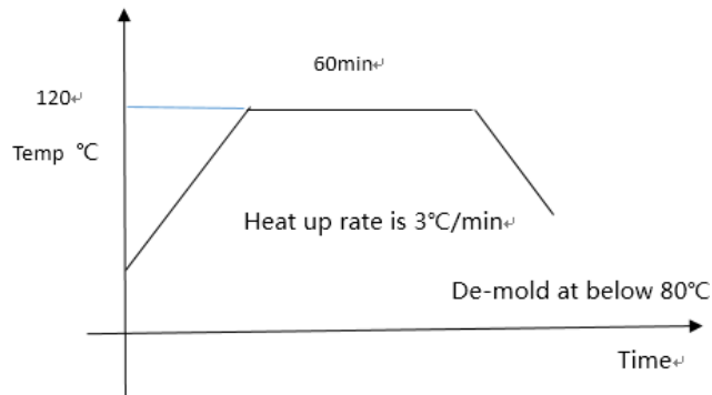
模具成型固化条件的一个例子
